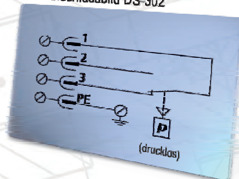
2. Anschlussbild DS-302
