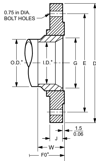
ANSI 150 # (CODE F0)
