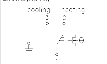
LR 80. .... (TR/TW)
