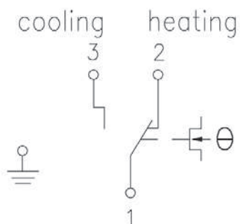
KR 80. .... (TR/TW)
