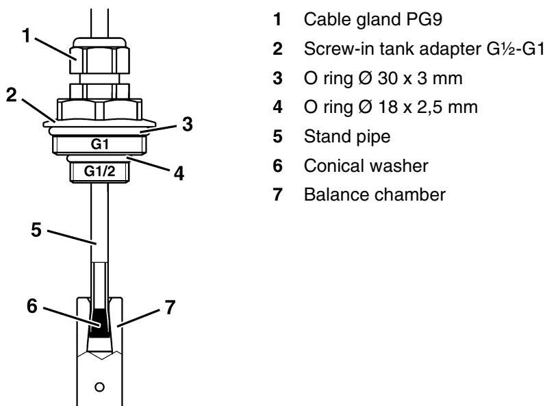
Fig. 2: Tubing kit
